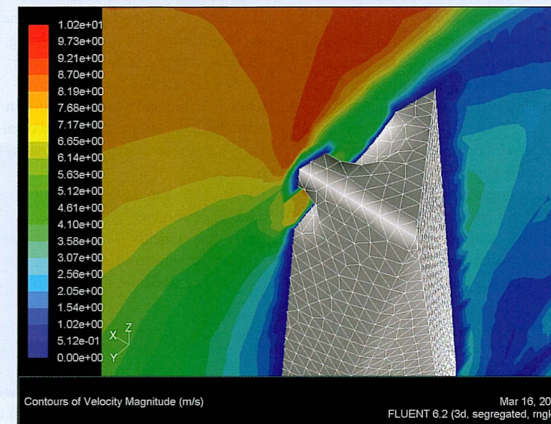
Contour plot van de snelheden in een verticaal vlak door een van de gaten van de Kite Tower. Wind loodrecht op de gevel, C gelijk aan 10.
