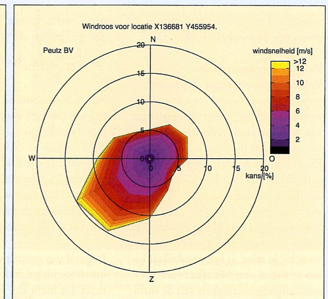
Windroos op 60 meter hoogte voor Scheveningen en Utrecht (bron data: NPR 6097). In de figuur is de kans op het voorkomen van wind uit een bepaalde windrichting en de verdeling van snelheden binnen die windrichting weergegeven.
