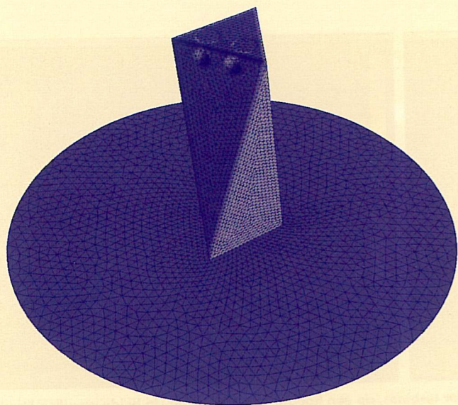
Gemodelleerde geometrie van de Kite Tower. Het gebruikte rekengrid op het oppervlak van de toren en de gemodelleerde windturbines is zichtbaar.
