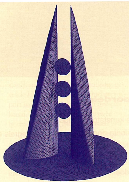
Gemodelleerde geometrie van het WTC te Bahrain. Het gebruikte rekengrid op het oppervlak van de torens en de gemodelleerde windturbines is zichtbaar.
